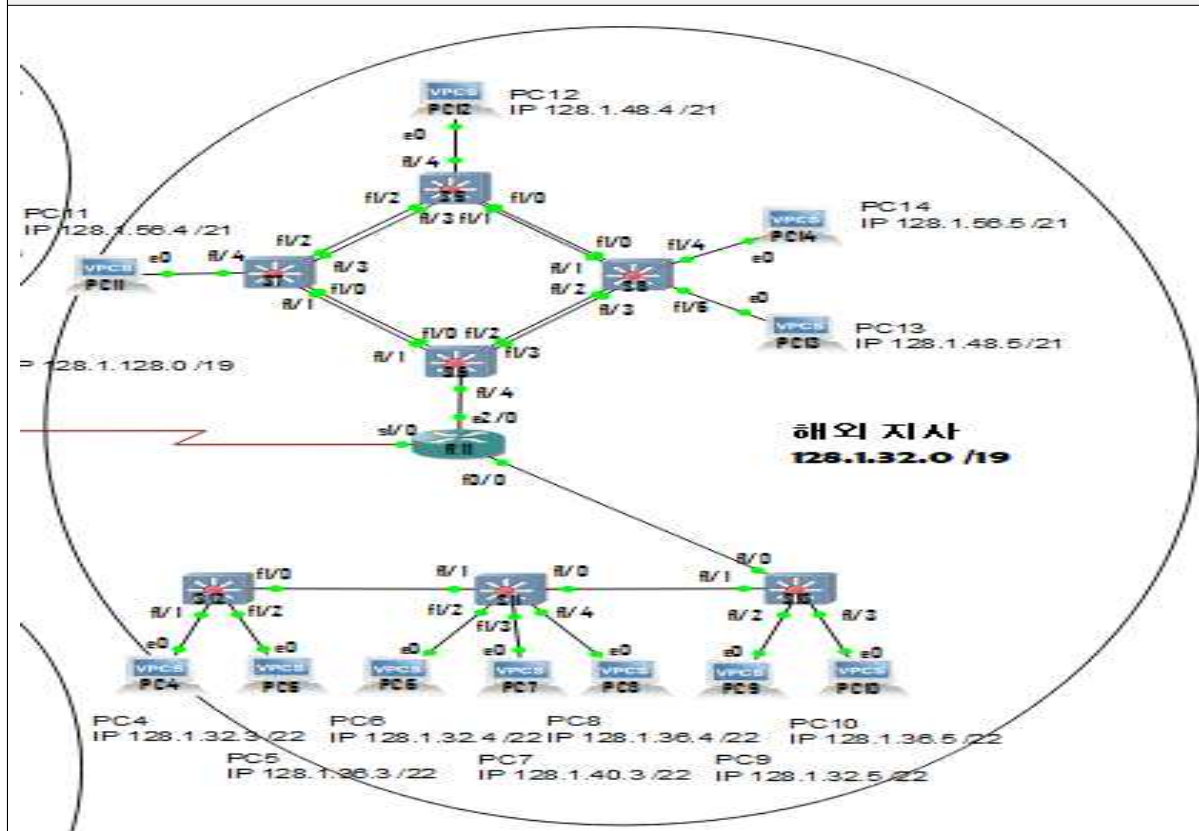
지사(L2)구역 상세 네트워크 구성도
